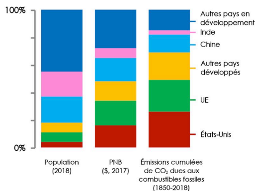
Population, richesse et émissions cumulées
